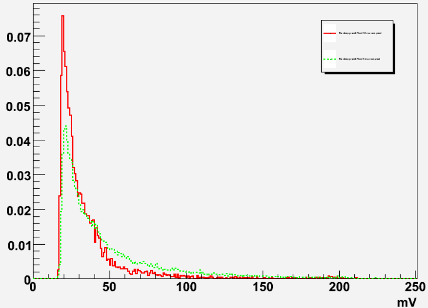
Fe55 Spectrum
