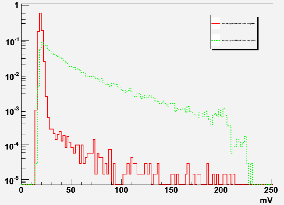
Fe55 Spectrum
