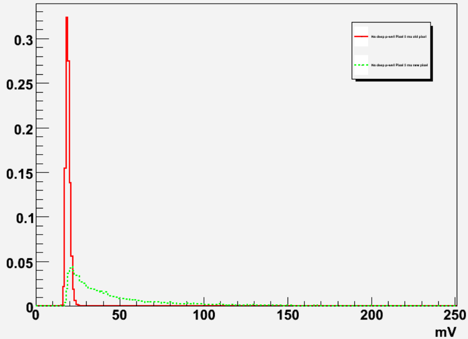
Fe55 Spectrum
