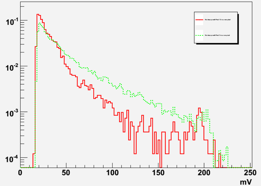
Fe55 Spectrum
